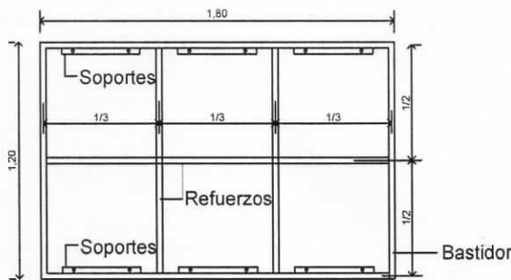
VISTA FRENTE BASTIDOR SIN CHAPA
