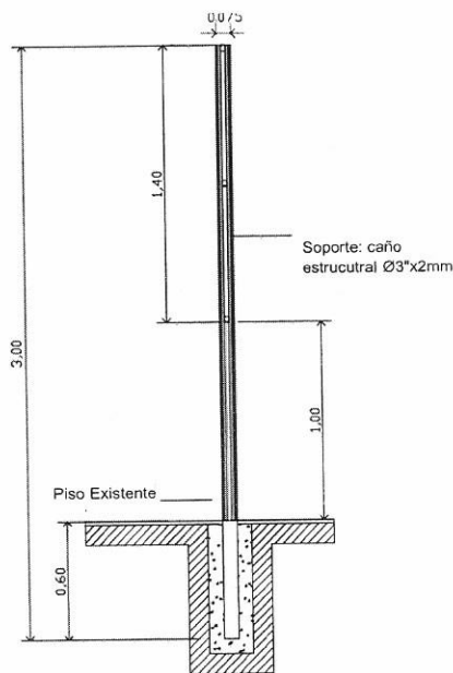
CORTE TRANSVERSAL
