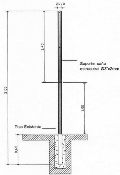
CORTE TRANSVERSAL
