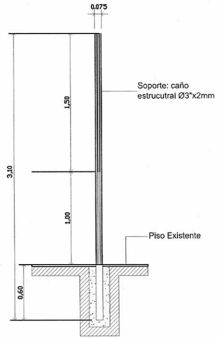
CORTE TRANSVERSAL
