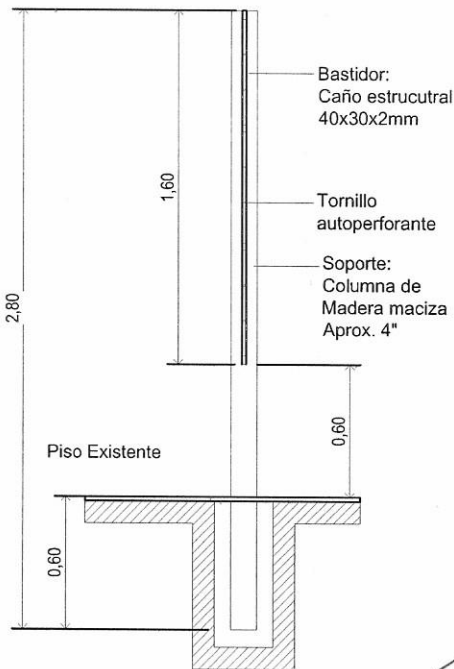
CORTE TRANSVERSAL
