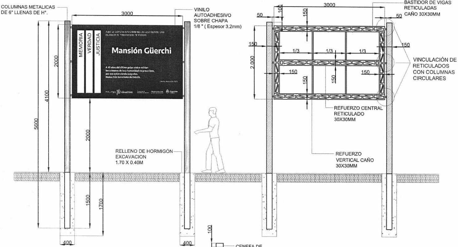
VISTA FRENTE CON CHAPA DE RECUBRIMIENTO
