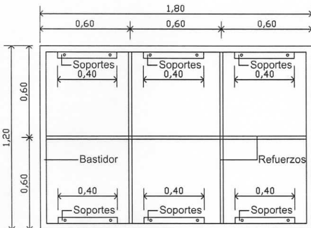
VISTA FRENTE BASTIDOR SIN CHAPA
