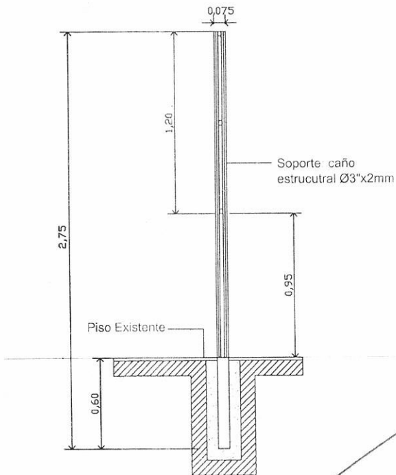
CORTE TRANSVERSAL
