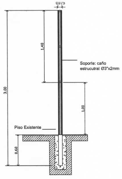
CORTE TRANSVERSAL
