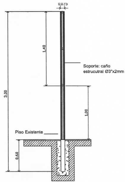
CORTE TRANSVERSAL
