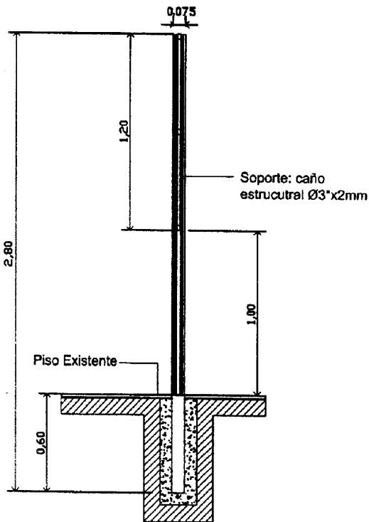
CORTE TRANSVERSAL
